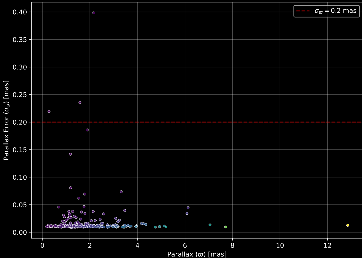
GALAH DR4 Field: [193] Parallax Quality (n= 300)
