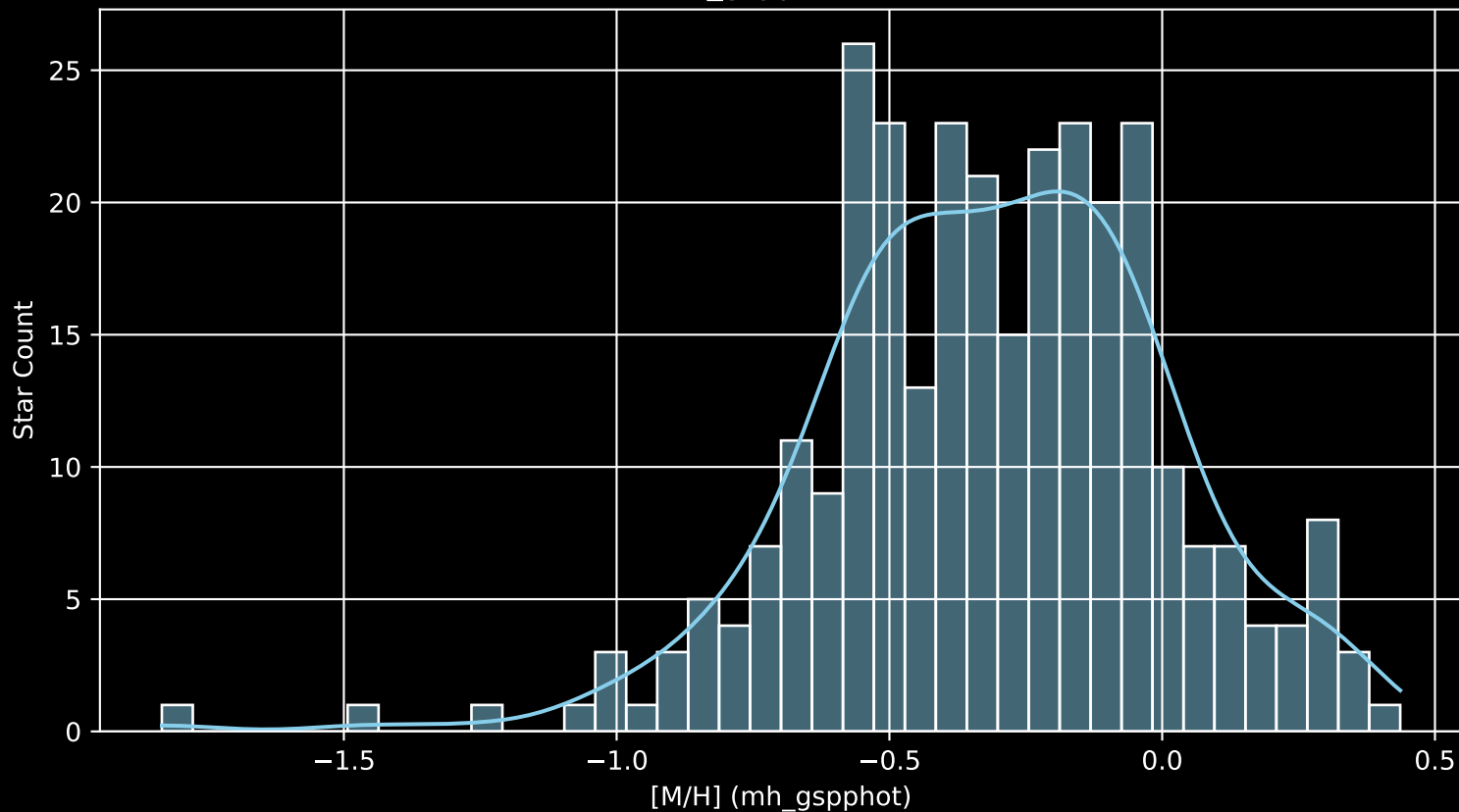
GALAH DR4 Field: [193] [M/H] (mh_gspphot) (n= 300)
