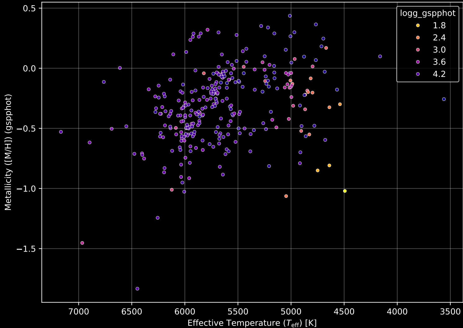
GALAH DR4 Field: [193] Stellar Population Parameters (n= 300)
