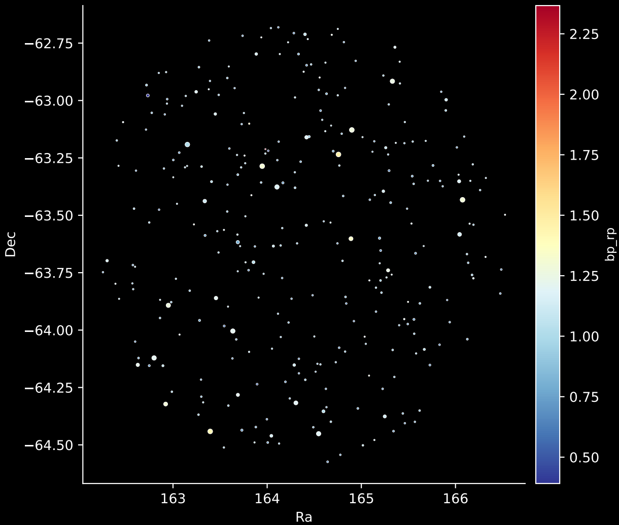
GALAH DR4 Field: [193] Stars: 300
